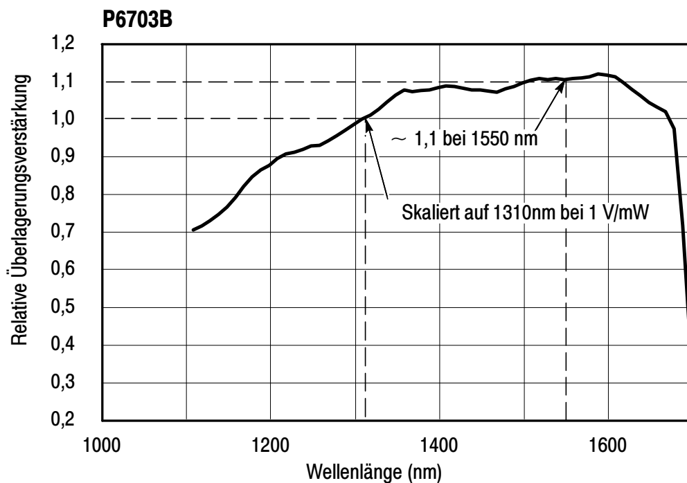
Abbildung 7: Typische wellenlängenabhängige Verstärkung (25° C Umgebungstemperatur)
