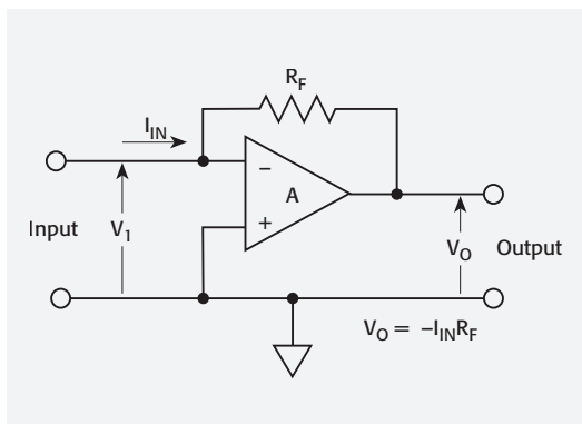
Feedback Ammeter
